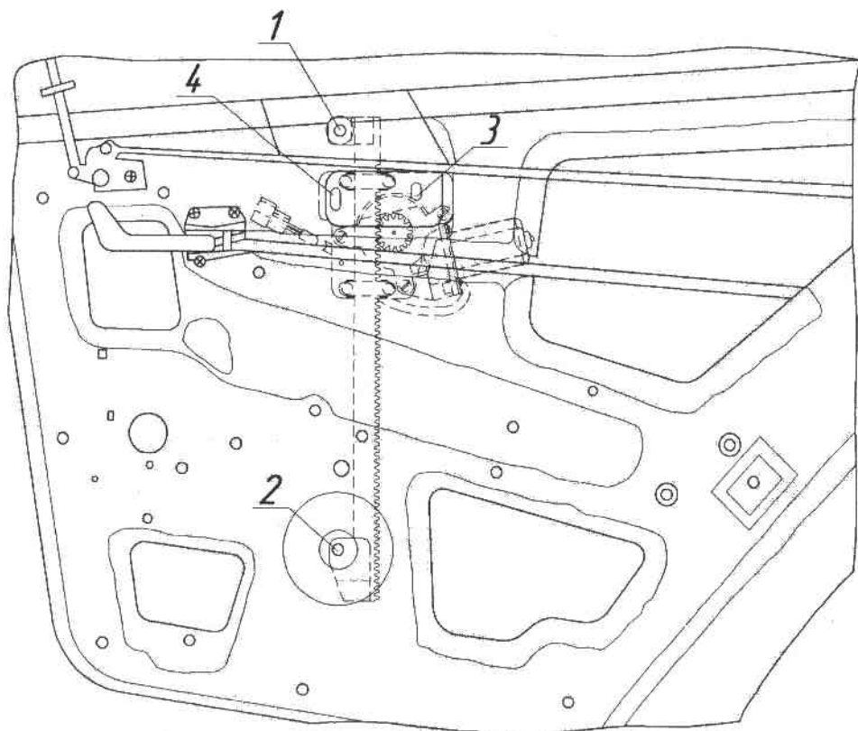
Установка ЭСП в заднюю правую дверь рис. 3
